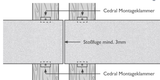
Ausbildung der Stoßfugen mit Cedral Montageklammern
