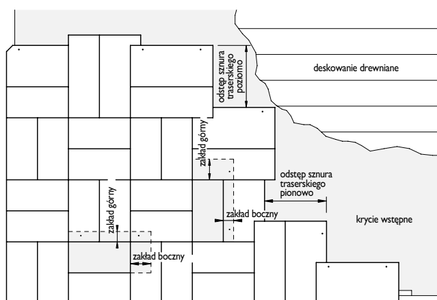
Krycie mozaikowe lewe, 40 x 20 cm, z docinanymi krawędziami szczytowymi
