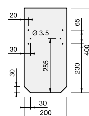
20 x 40 cm, ze ściętymi rogami
