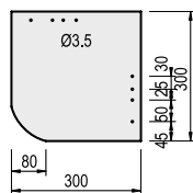
30 x 30 cm, zaokrąglone
