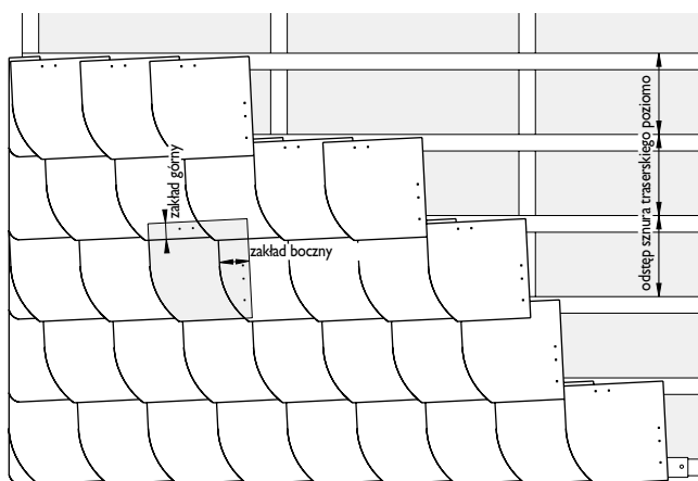
Przykład: Format 30 x 30 cm, cięcie łukowe lewe, ze zintegrowanym szczytem początkowym
