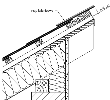
Kalenica pulpitowa na deskowaniu
