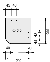
20 x 20 cm, zaokraglone
