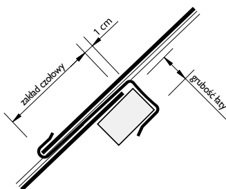
Mocowanie hakiem typu H
