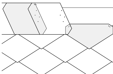
Krycie kalenicowe z obróconymi płytkami dachowych oraz rząd płytek kalenicowych
