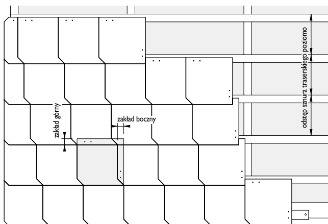
Przykład: Format 30 x 30 cm, ze ściętymi rogami, z docinającym kryciem szczytu
