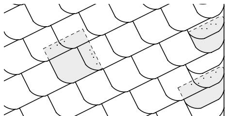
Wykończenie krawędzi szczytowej w sposób podwójny
