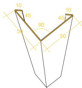
Perfil esquinero
