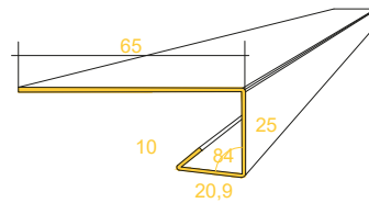
Corta gotera ventana
