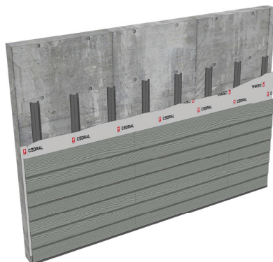
Revestimiento de fachada sobre hormigón
