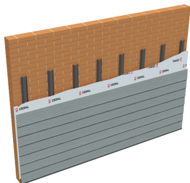
Revestimiento de Fachada sobre ladrillo
